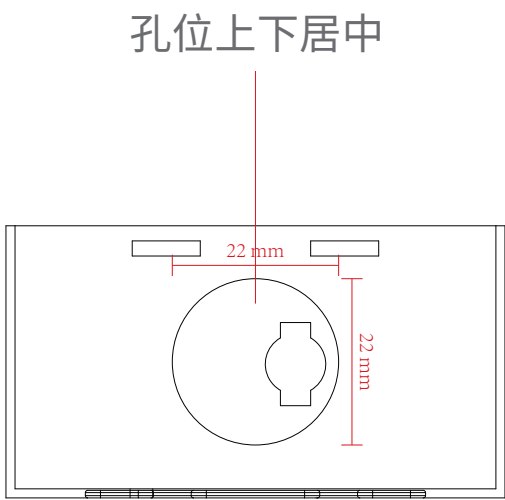
右视图
