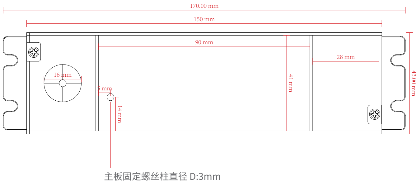
顶视图
