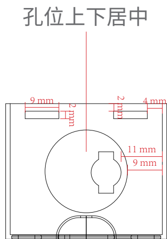
左视图
