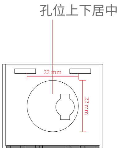
右视图
